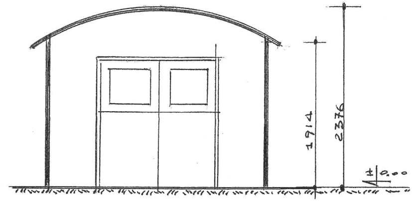
SEZIONE A-A
